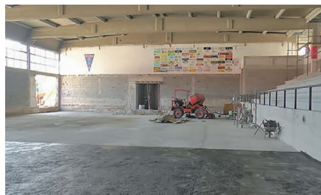
Реновирање хале у Чајетини
