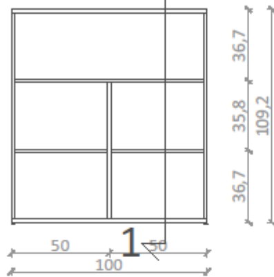
Izgled 1
